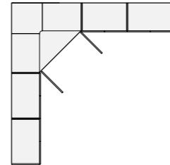
ANGOLO SPOGLIATOIO 45° DRESSING CORNER 45°
